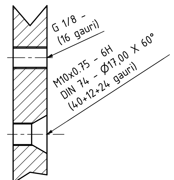
C-C ( 1 : 1 )
