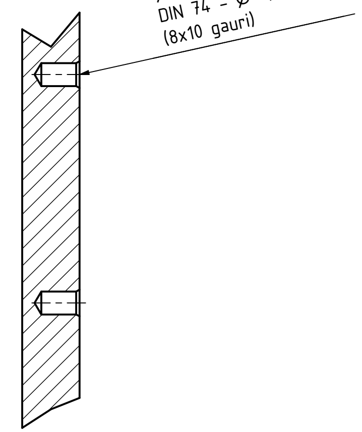
B-B ( 1 : 1 )
