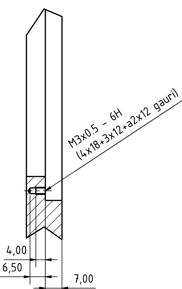
D-D ( 1 : 1 )
